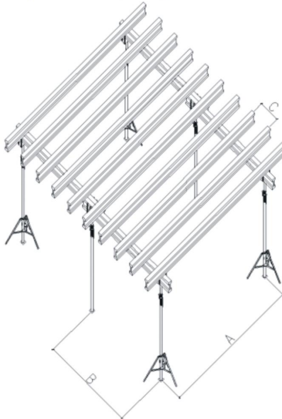
Схема растановки опалубки перекрытий
